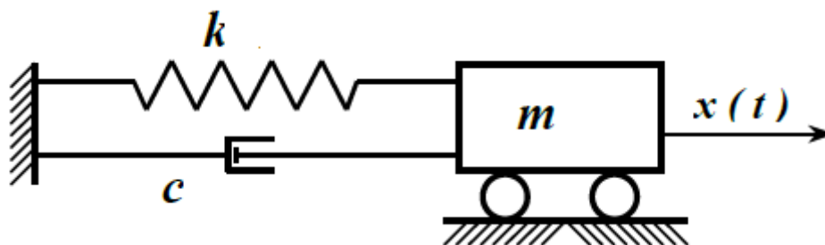
Figure 4.4: Système masse ressort amortisseur
