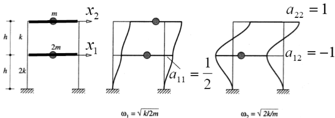
Figure 4.7: Cadre à deux degrés de liberté
