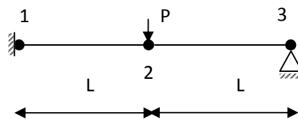
Figure 5.7: Poutre avec deux éléments
