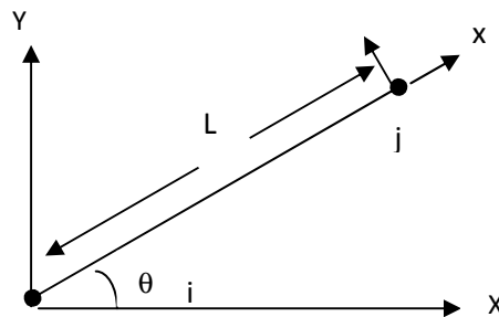
Figure 5.4 : Élément d'un treillis
