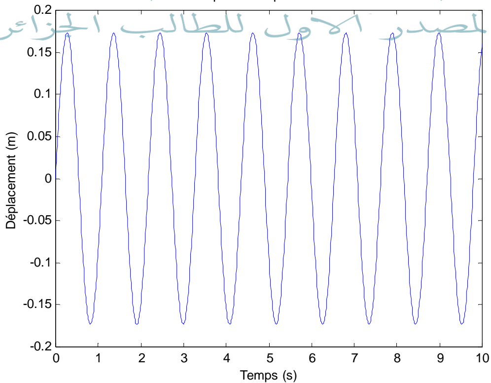
Figure 4. 3: Réponse temporelle libre
