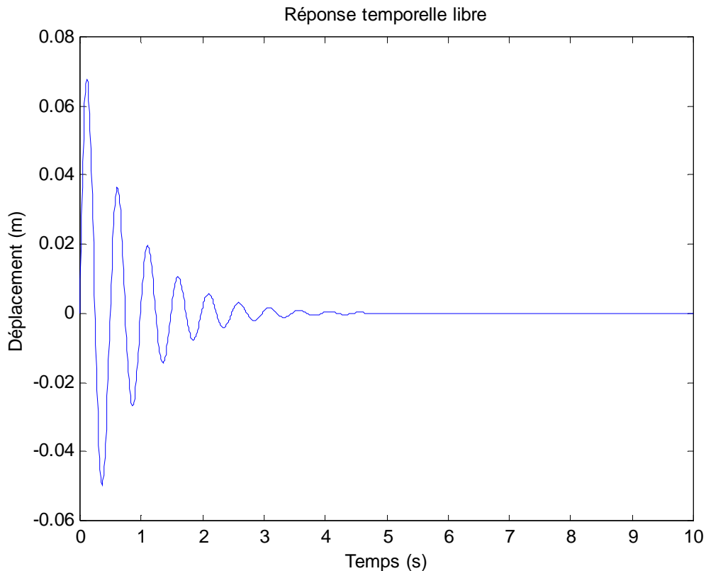
Figure 4.6: réponse temporelle libre amortie
