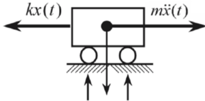
Figure 4.2: Forces présentes dans un système non amorti
