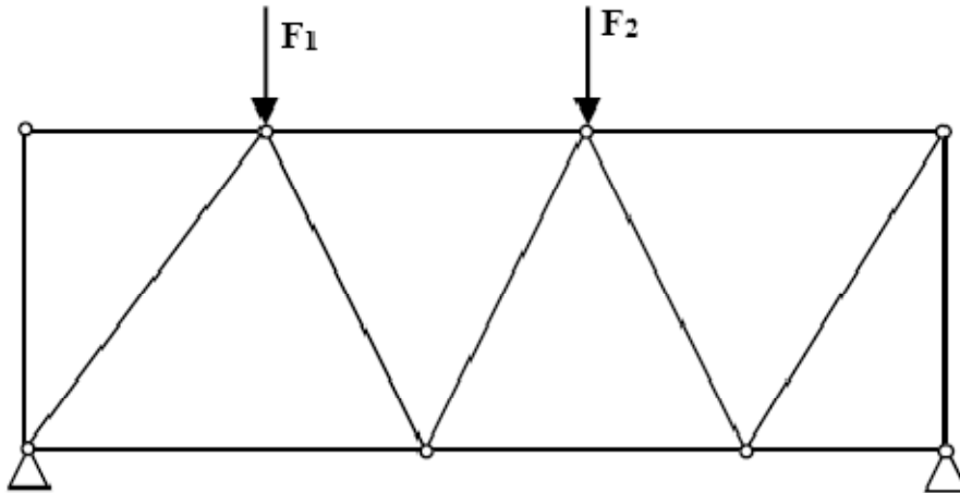
Figure 5.3 : Système à treillis
