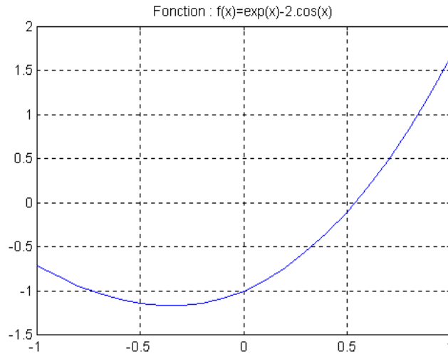
Figure III.1 : Localisation de la valeur x_0 où f(x_0) \approx 0
