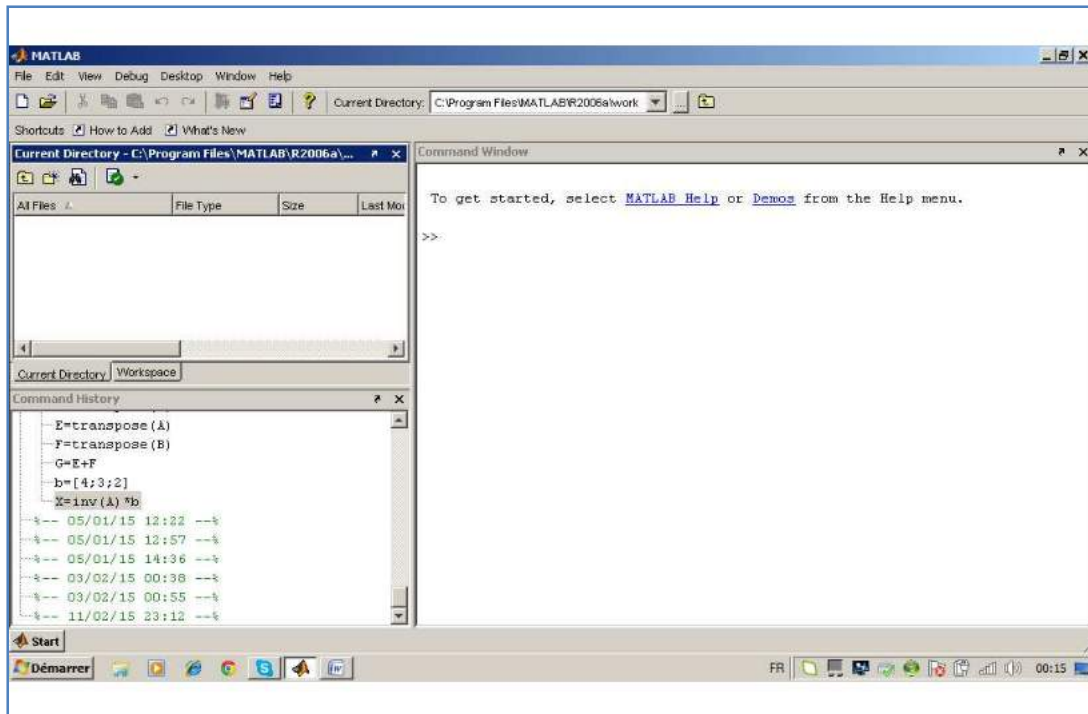
Figure I.1 : L'environnement MATLAB
